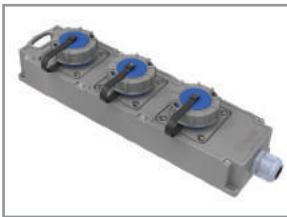
BG6-1010-1010 1/16A. 220V. 3 Pcs. IP67
