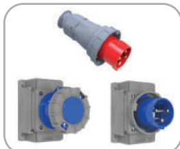
CEE Norm 16A. 24V. B
